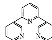
2,2',2''-terpyridine (terpy)
